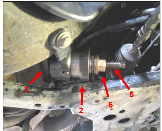
Einbau
